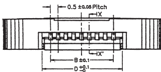
P.C.B. LAYOUT
