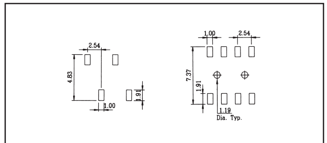
P.C.B. LAYOUT
