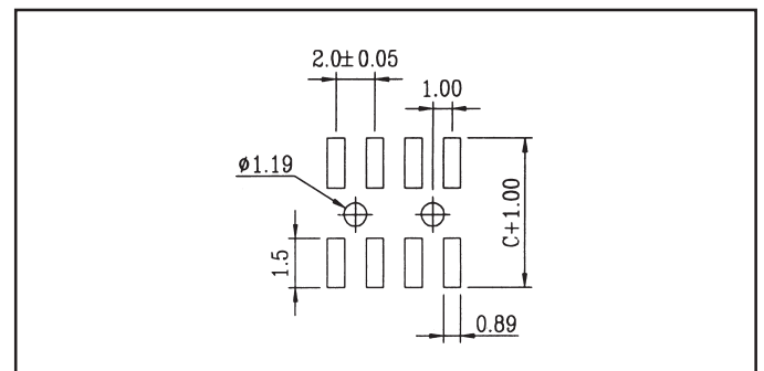
P.C.B. LAYOUT
