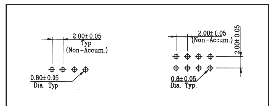
P.C.B. LAYOUT
