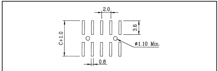
P.C.B. LAYOUT
